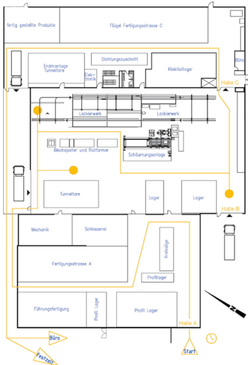
GRUNDRISS DES BATOR-FIRMENGEBÄUDES
